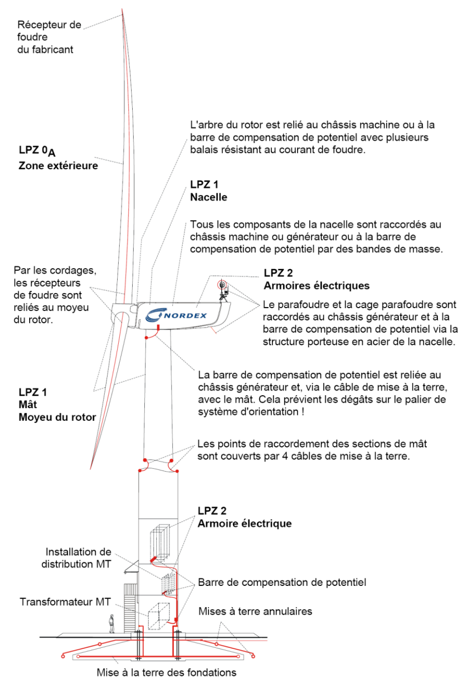
Figure 11 : Vue d'ensemble des dispositifs de protection parafoudre - NORDEX N131 (source : Nordex, 2018)
