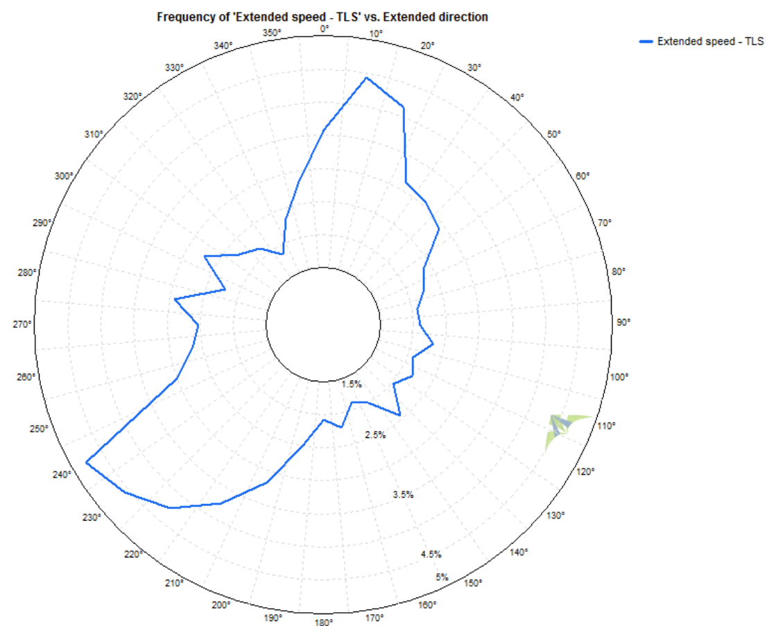
Figure 6 : Rose des vents (source : RWE, 2020)
