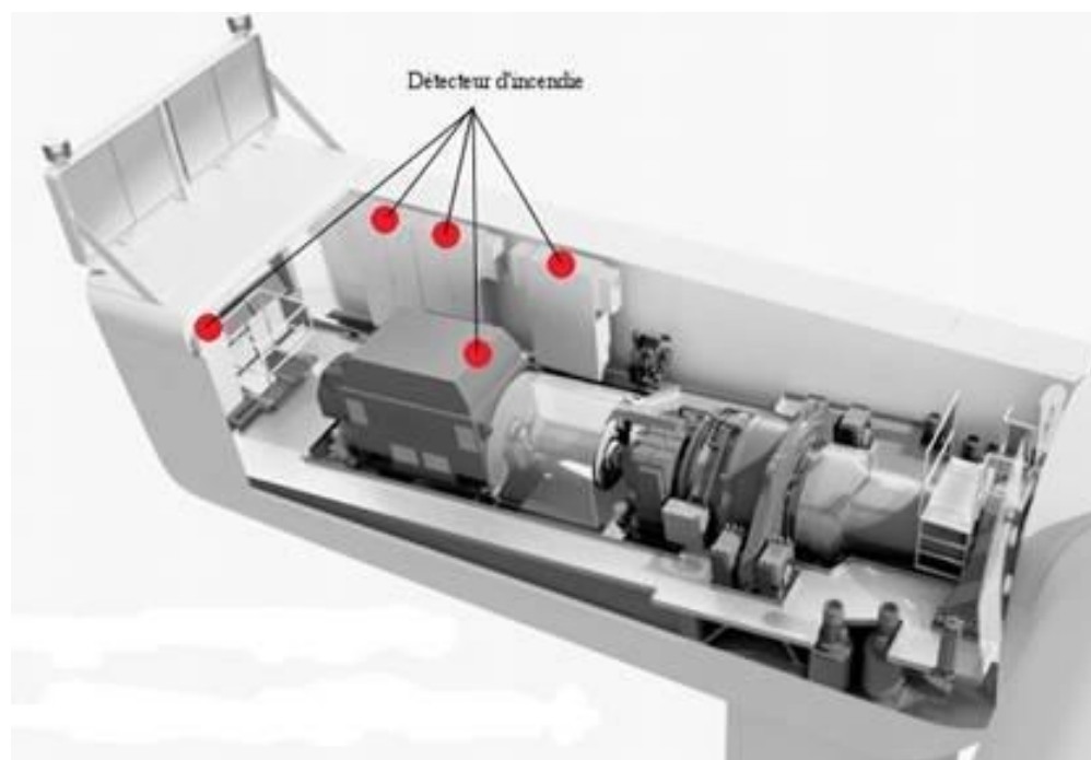
Figure 10 : Positionnement des détecteurs d'incendie dans la nacelle NORDEX N131 (source : Nordex, 2018)
