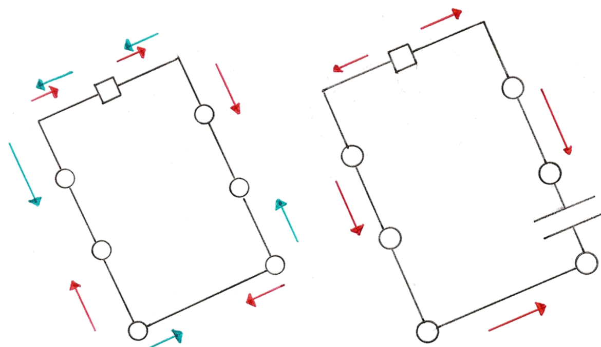
Figure 12 : Illustration du système en anneau garantissant une communication continue des éoliennes – Légende : ○ Eolienne □ SCADA → Circulation de l'information
